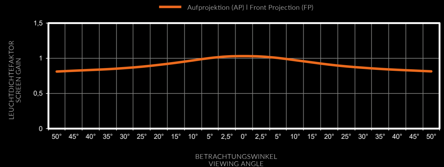
LEUCHTDICHTEFAKTOR NACH DIN 19045 | GAIN ACCORDING TO DIN 19045 FLEX WHITE BLACK MOX
